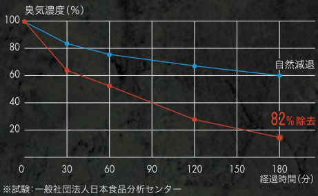
<アンモニアに対する除去性能>
